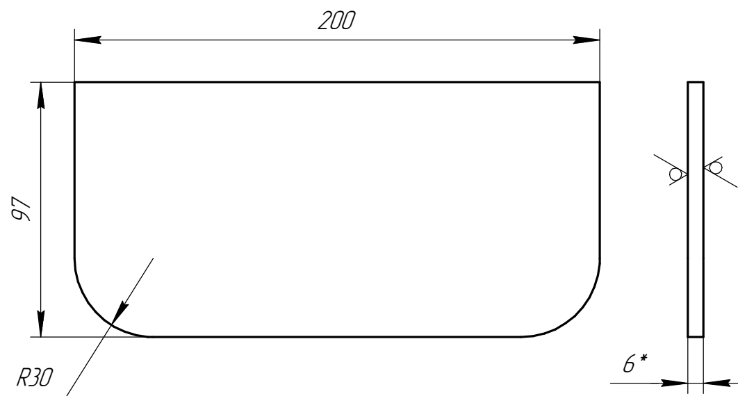
Дет. поз. 2 (1:2)
