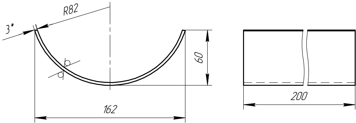
Дет. поз. 1
