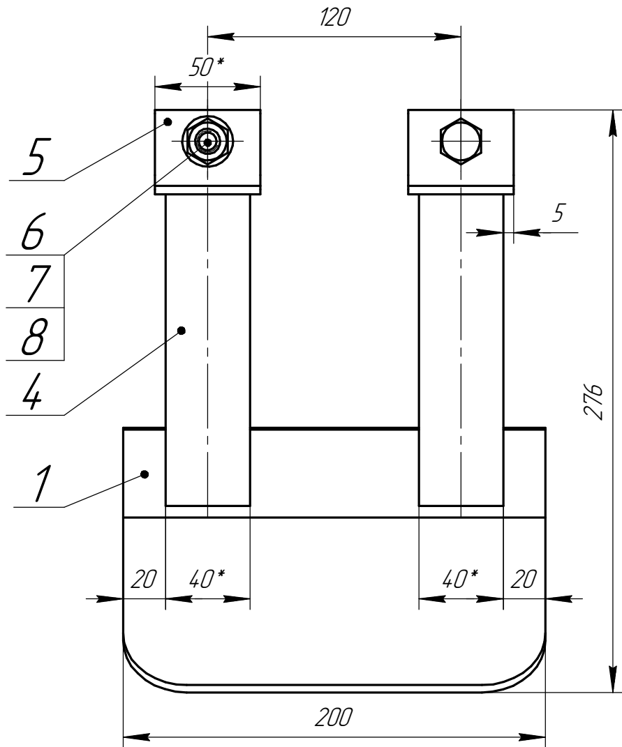
Дет. поз. 3
