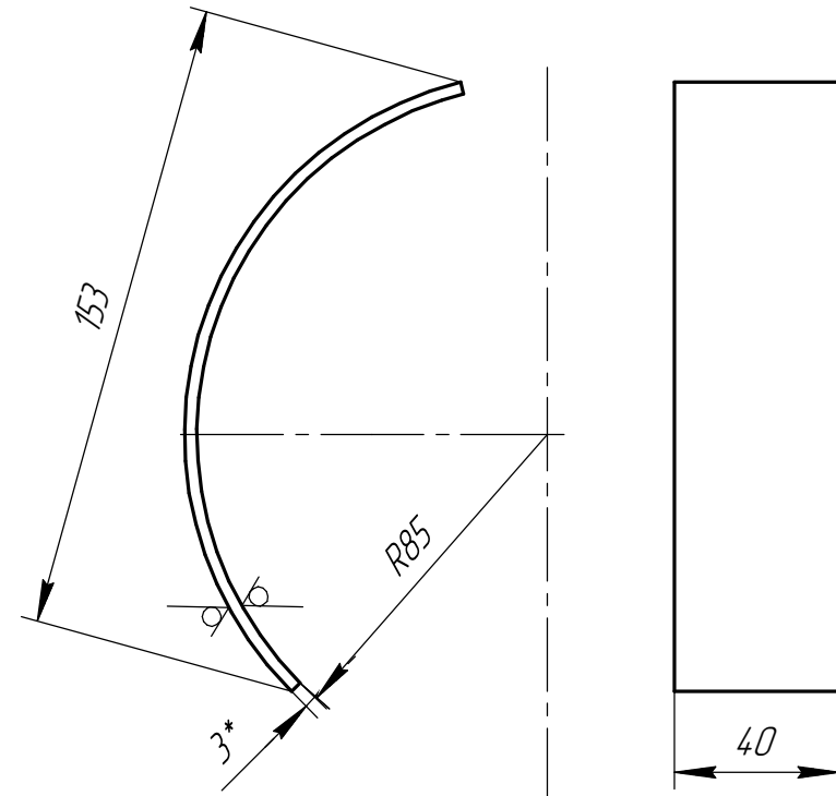
Дет. поз. 4 (1:2)
