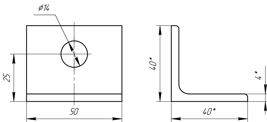
Дет. поз. 5 (1:1)
